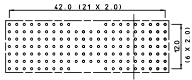
LAY-OUT P.C.B. - HOLE
